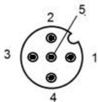
5 POLIG / 5-pole
