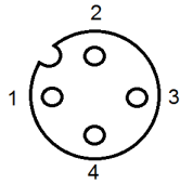
4 POLIG / 4-pole
