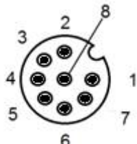
8 POLIG / 8-pole
