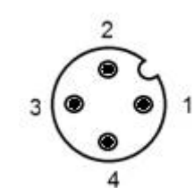
4 POLIG / 4-pole
