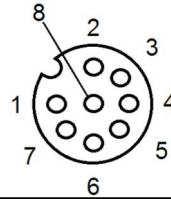
8 POLIG / 8-pole
