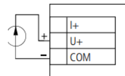
Spannungssignal / voltage sensor wiring
