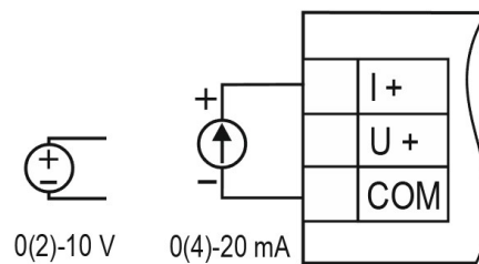
Fig. 5.5 Input wiring
