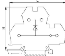
Nq4-Diode V3
