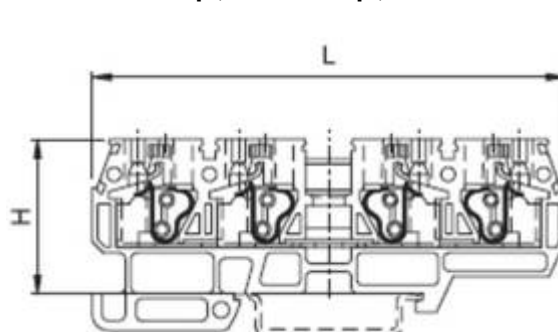
Euro QM 2/2-2,5/35 Nq2,5-2-G & Nq2,5-2-BL
