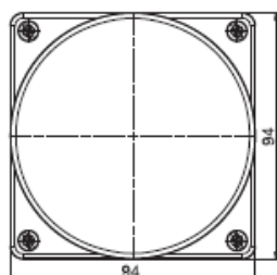
Gehäuse / case
