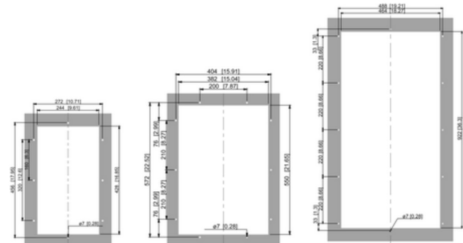
TG 6155 / 6205 / 6255 Anbau
