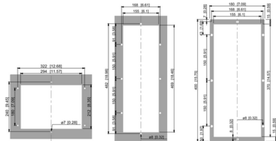
TG 6105 Anbau
