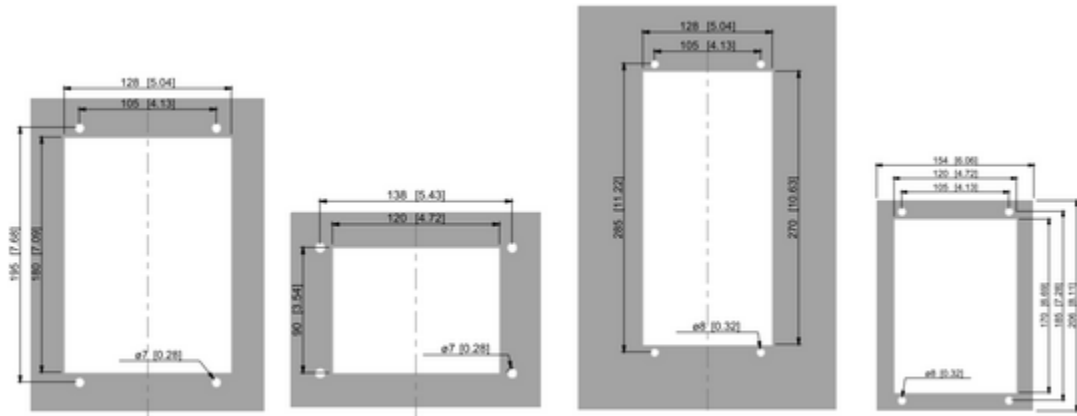
TG 3030 Anbau
