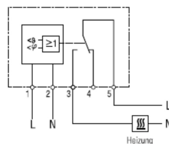
Anschlussdiagramm
