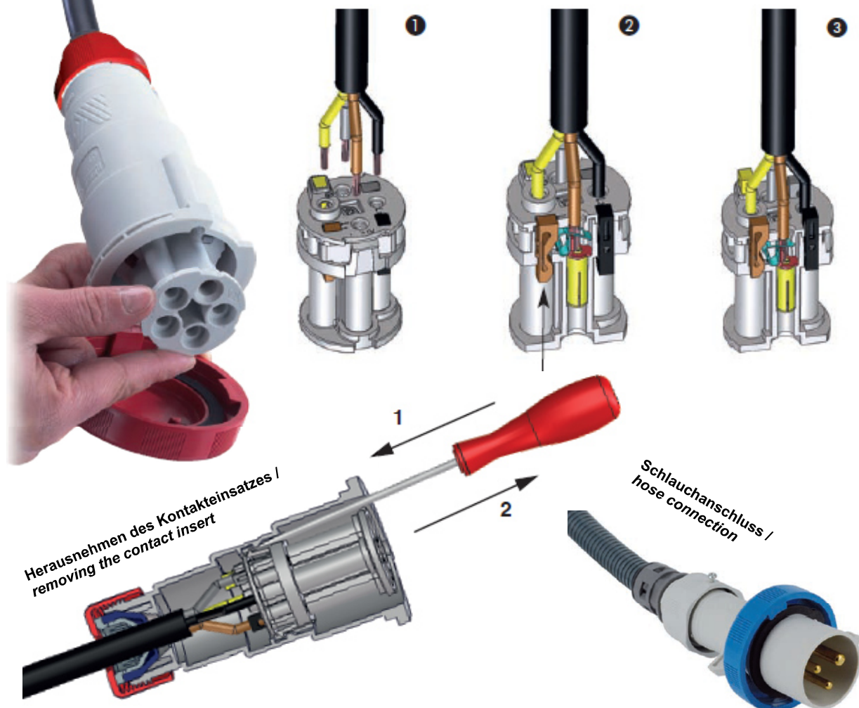
Anschlussprinzip
