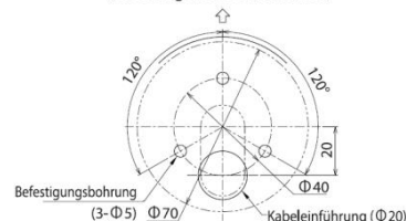
Produktvorderseite (Richtung des Schallaustritts)
