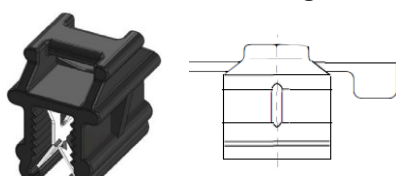
Oben rechtwinkelig
