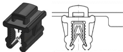
Oben längs
