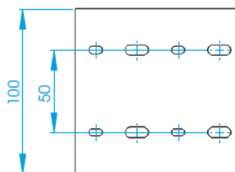
VK 100mm Breite/Width/Largeur
