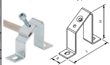
Montageclip für Kupferschienen / mounting clip for copper rails
